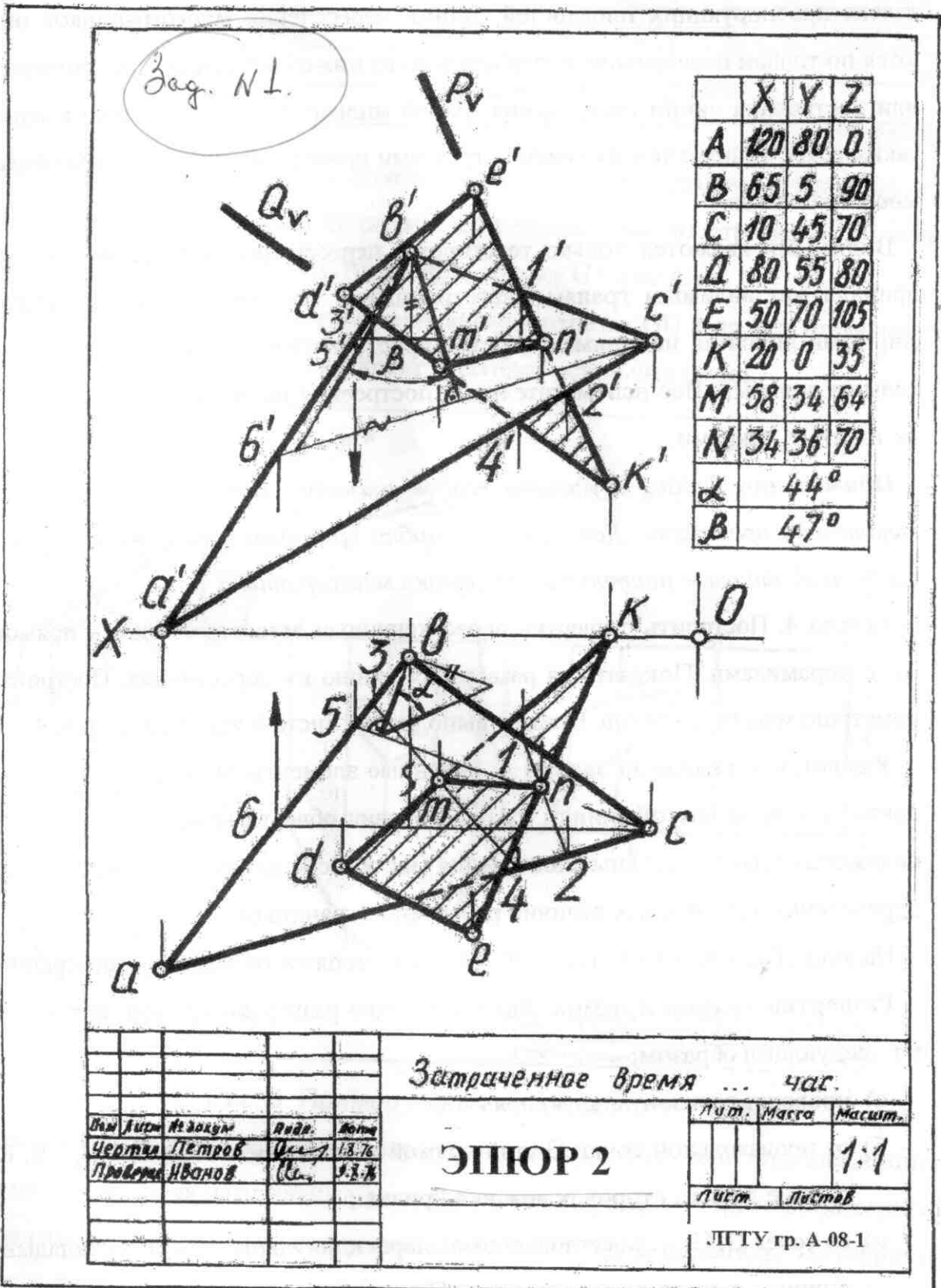
Рис. 2. Пример выполнения листа 2
